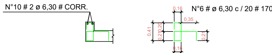
VIGA VA - 20 x 45 cm (2X)
