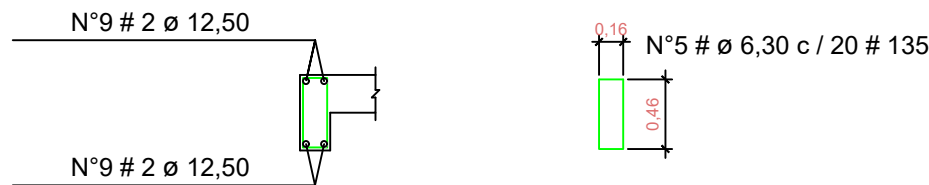
VIGA VB (2X)
