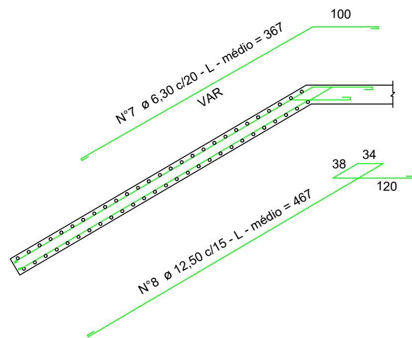
CORTE B - B ESC 1:25
